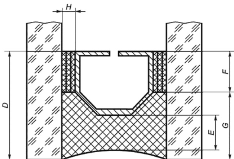
Рисунок 2 - Герметизирующие слои стеклопакета
