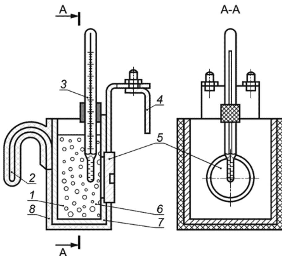
Рисунок 7 - Схема прибора с контактной латунной пластиной для контроля точки росы
