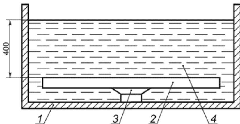
Рисунок А.1 - Схема испытательного стенда
