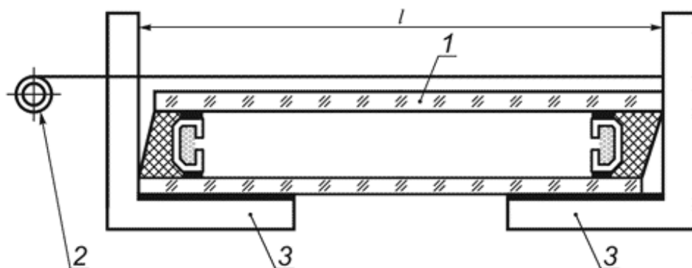
Рисунок 4 - Измерение высоты (длины), ширины стеклопакета
