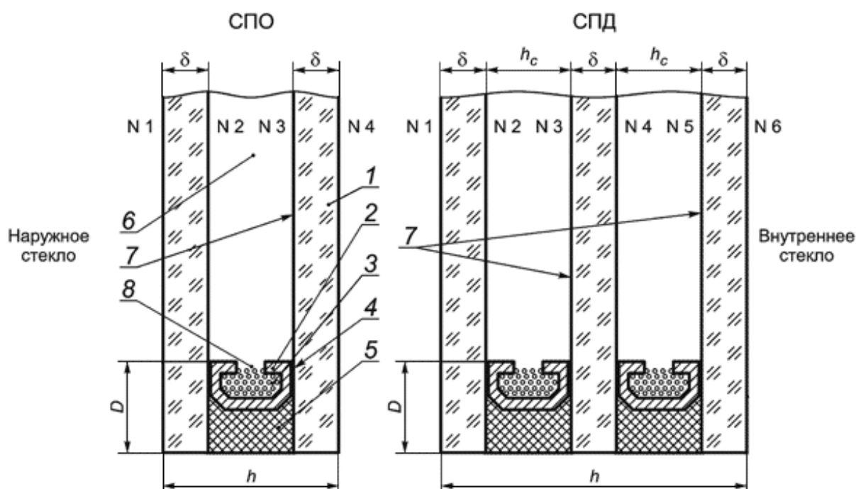
Рисунок 1 - Типы и конструкции стеклопакетов
